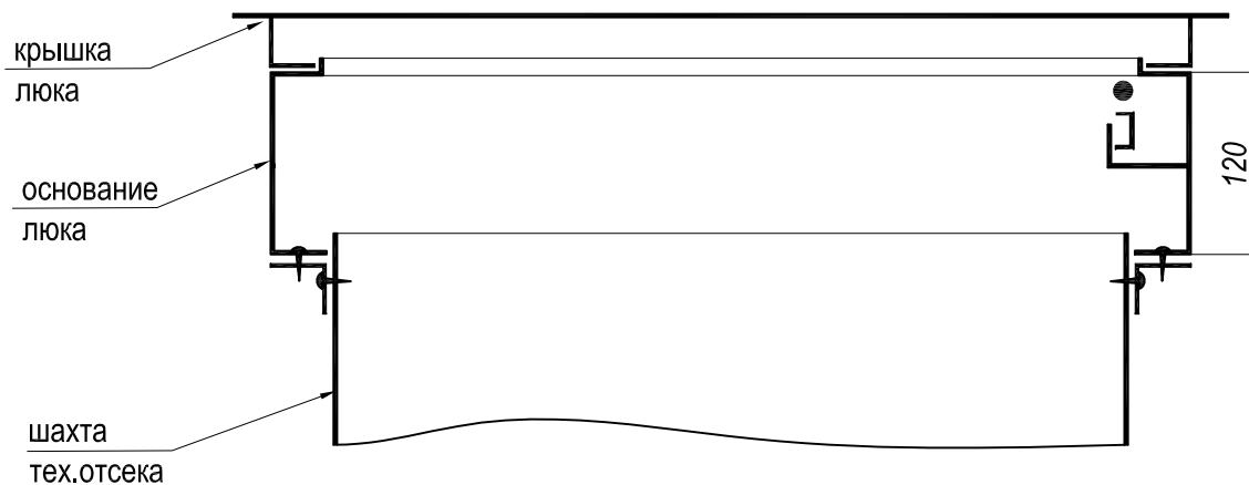
A-A (вариант 2)
